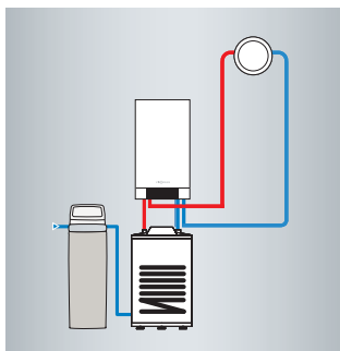
Príklad vykurovacieho systému s plynovým kotlom a stanicou na úpravu vody.
